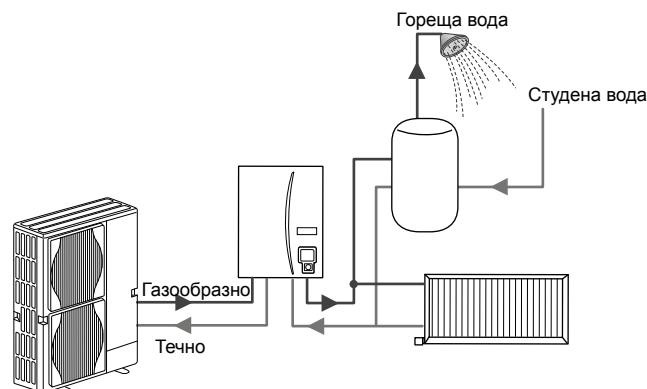
Изображение на термopомпенната система с Hydrobox
