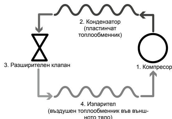
Изображение на термopомпенната система с Hydrobox
