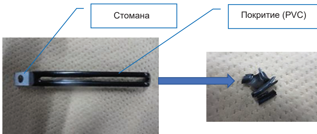
Фиг. 1 Клема
